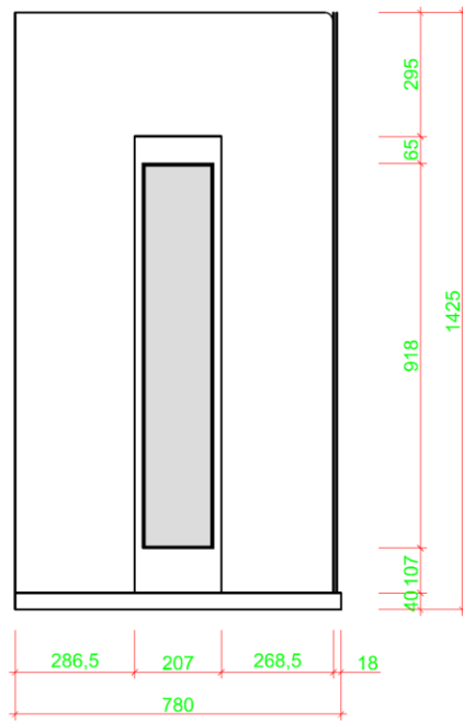
Ansicht Vorderwand
