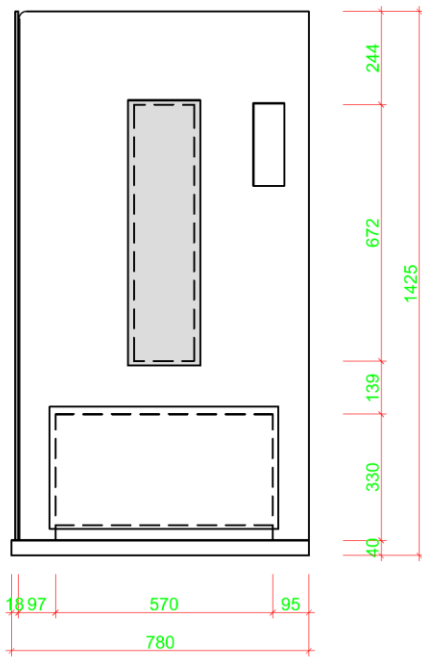
Ansicht Rückwand
