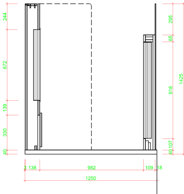
Vertikalschnitt
